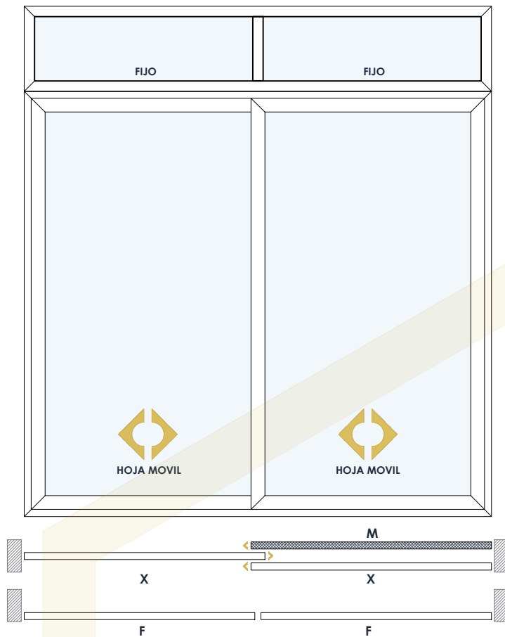
CORREDIZA + FIJO 2 HOJAS MOVILES + 1 MOSQUITERO
