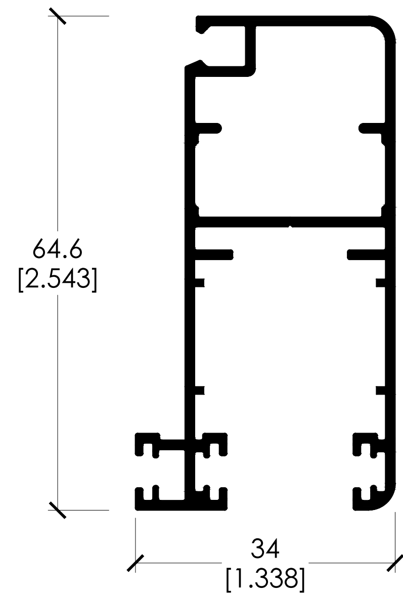
CLAVE: 2023 HOJA PERIMETRAL MOSQUITERO
