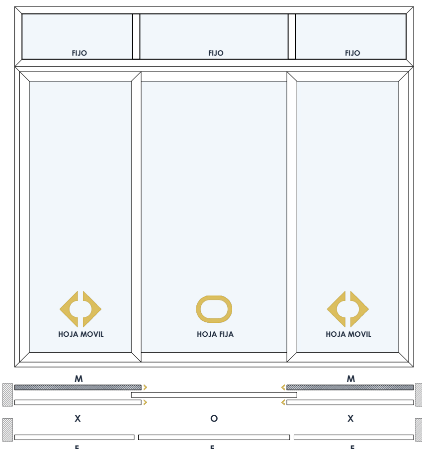
CORREDIZA + FIJO 2 HOJAS MOVILES + 1 HOJA FIJA + 2 MOSQUITEROS
