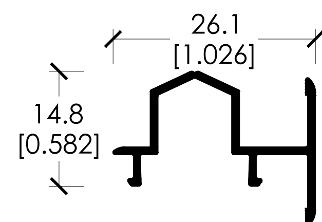
CLAVE: 2024 ADAPTADOR OXXO
