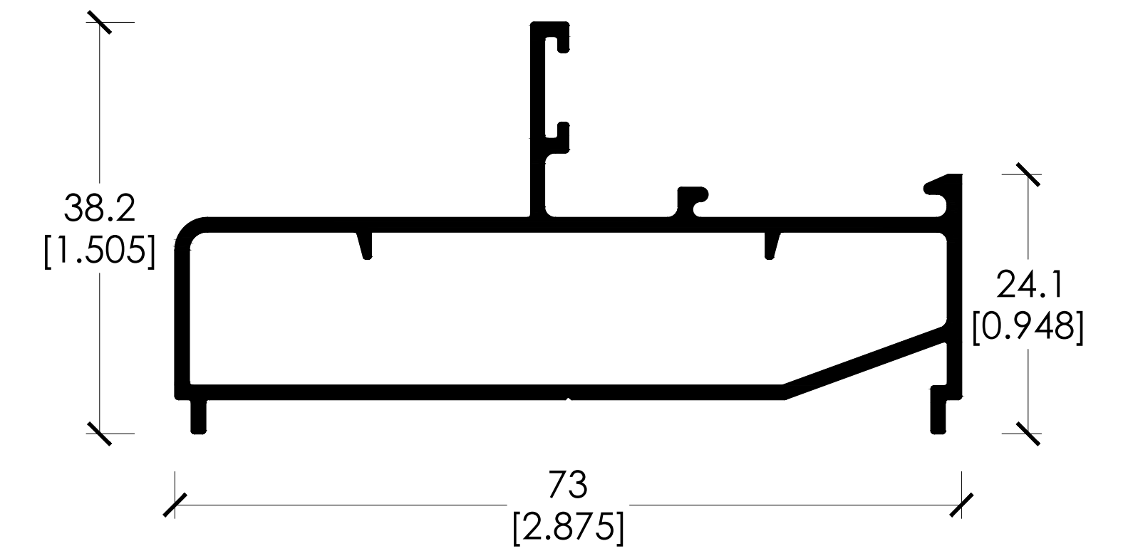
CLAVE: 2025 FIJO PERIMETRAL DOS VIAS
