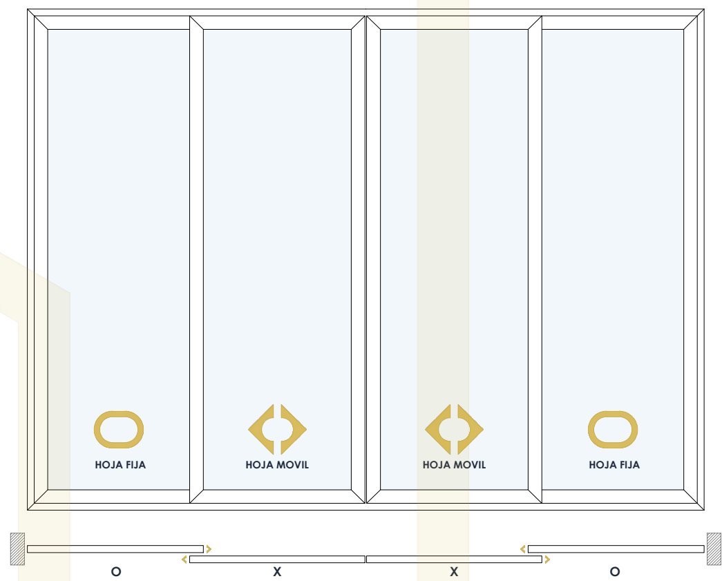
CORREDIZA 2 HOJAS MOVILES + 2 HOJAS FIJAS
