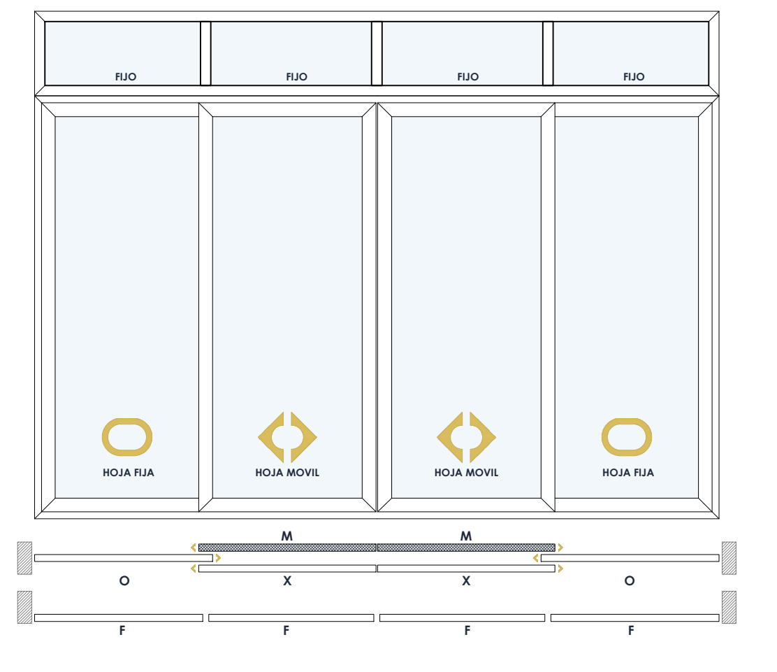
CORREDIZA + FIJO 2 HOJAS MOVILES + 2 HOJAS FIJAS + 2 MOSQUITEROS
