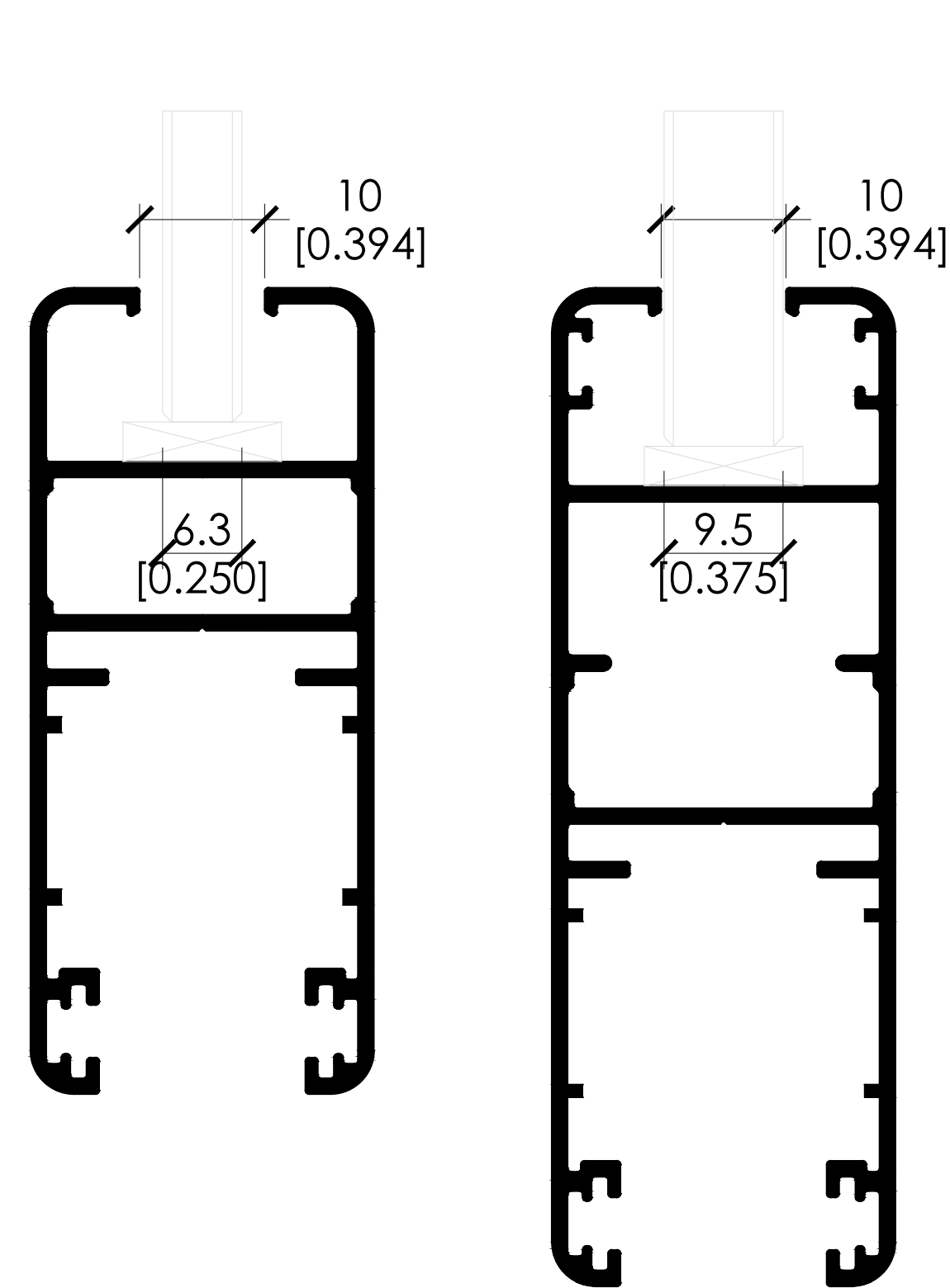
CLAVE: 2018 HOJA PERIMETRAL
