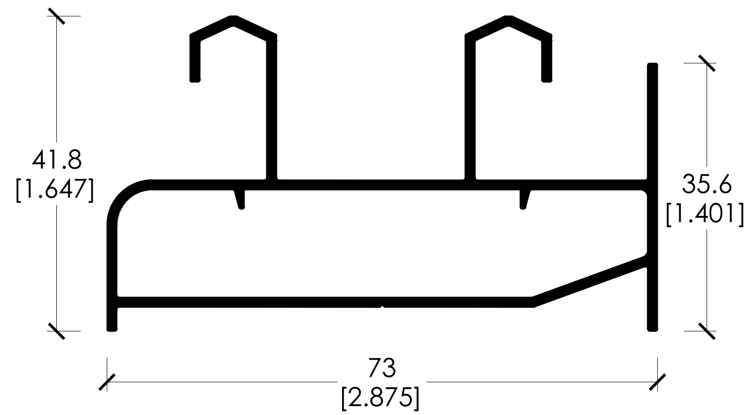
CLAVE: 2017 MARCO PERIMETRAL DOS VIAS
