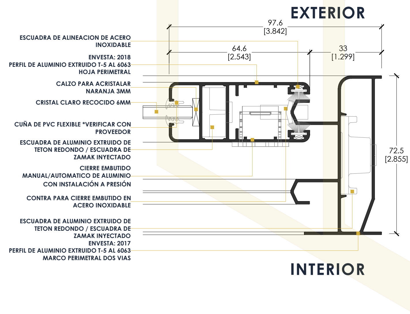
B-3 LATERAL CON CIERRE DE PRESIÓN
