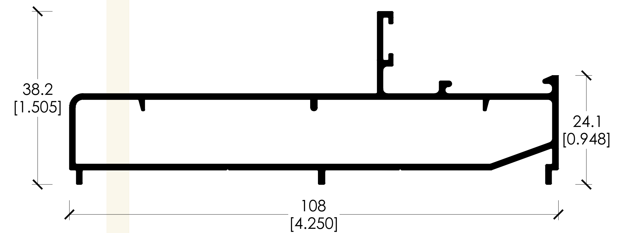
CLAVE: 2026 FIJO PERIMETRAL TRES VIAS
