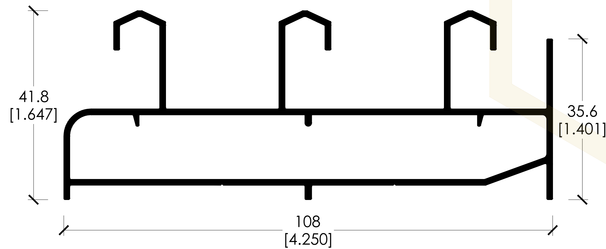
CLAVE: 2020 MARCO PERIMETRAL TRES VIAS
