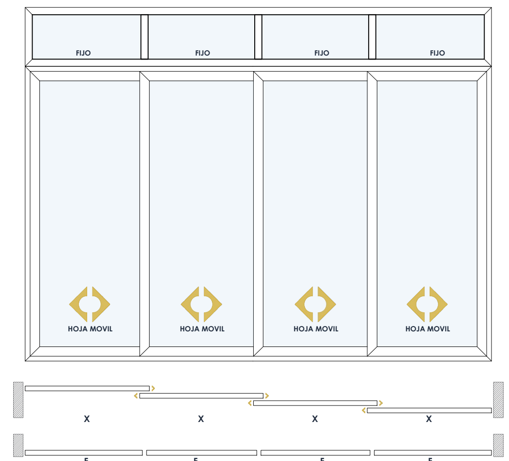
CORREDIZA + FIJO 4 HOJAS MOVILES
