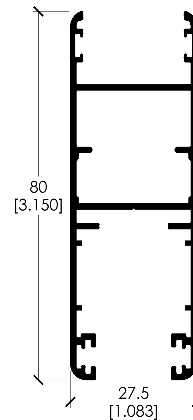
CLAVE: 2029 HOJA PERIMETRAL EURO 80 DOBLE VIDRIO
