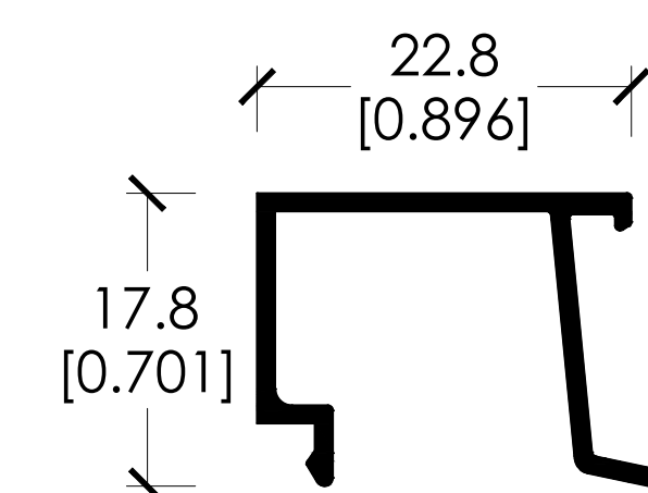
CLAVE: 2010 JUNQUILLO 9 a 12 mm
