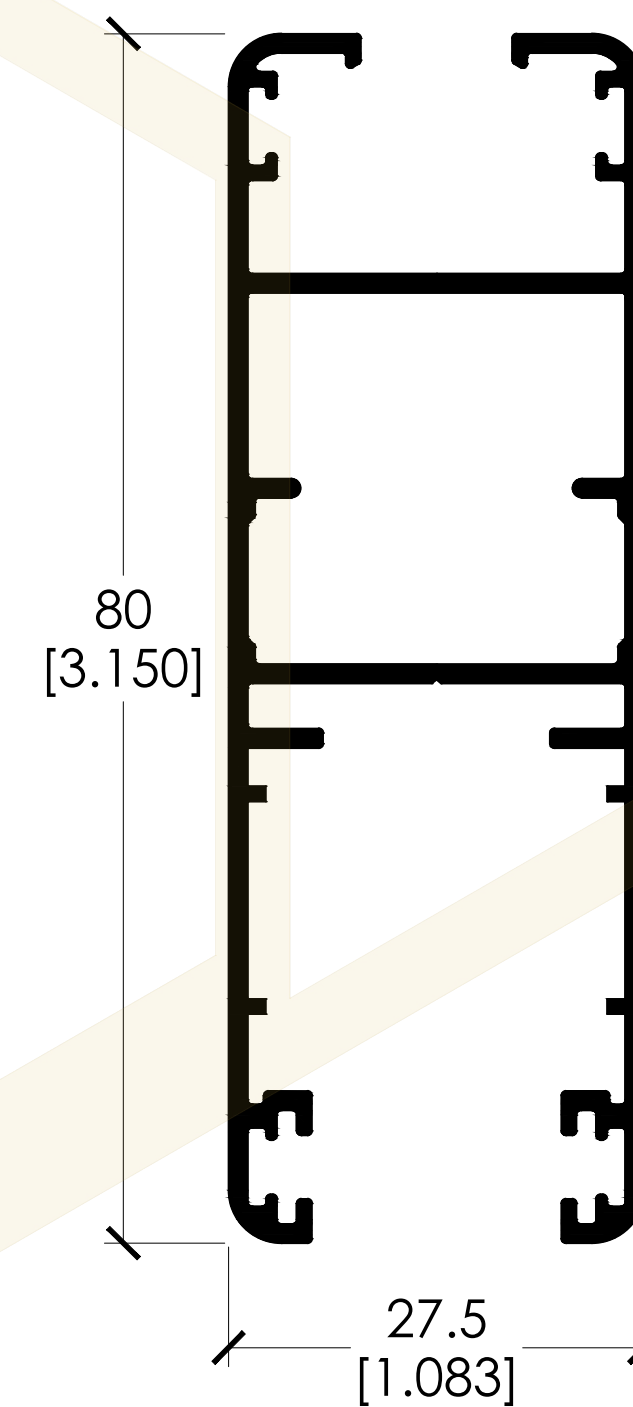
CLAVE: 2027 HOJA PERIMETRAL EURO 80
