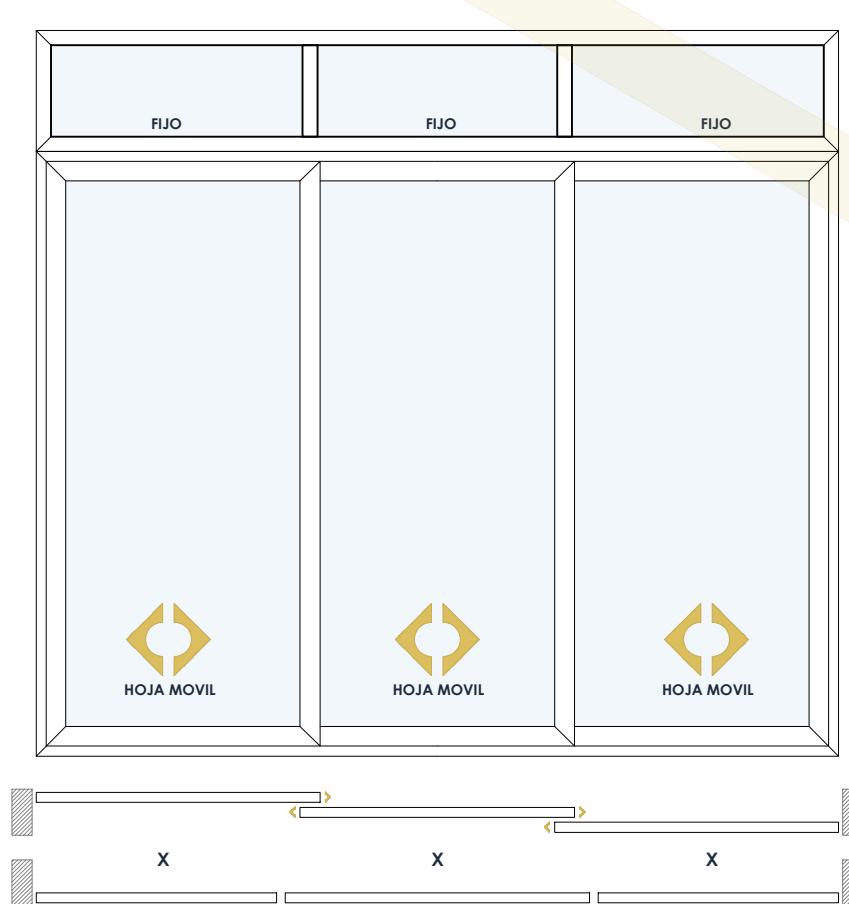
CORREDIZA + FIJO 3 HOJAS MOVILES
