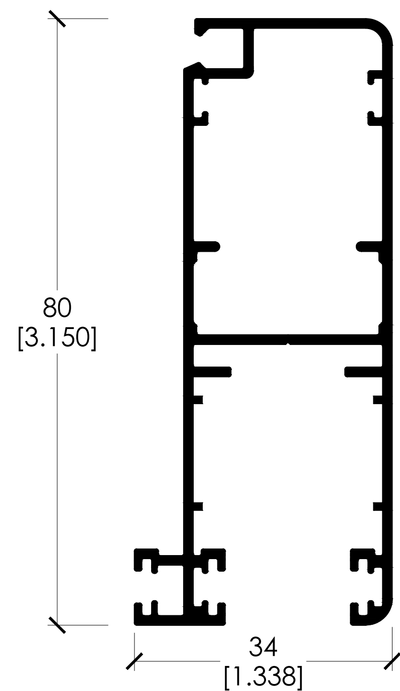
CLAVE: 2030 HOJA PERIMETRAL EURO 80 MOSQUITERO
