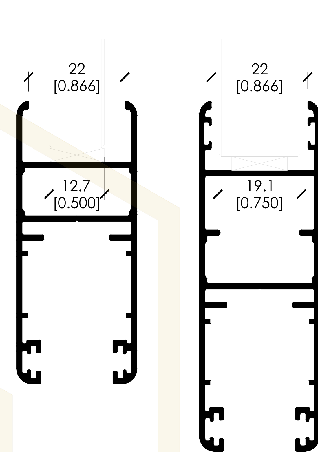
CLAVE: 2022 HOJA PERIMETRAL DOBLE VIDRIO
