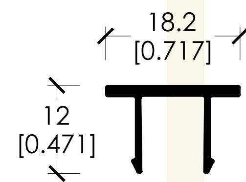
CLAVE: 2032 TAPA TIRADOR REFUERZO
