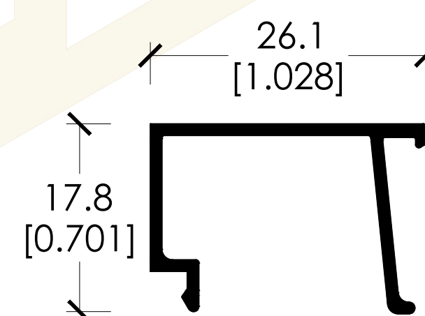
CLAVE: 2009 JUNQUILLO 6 a 9 mm
