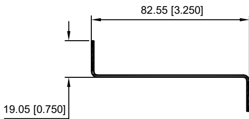
10002—PERFIL Z 3 1/4 LIGERO
