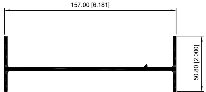
10013—PERFIL I PERALTE 6
