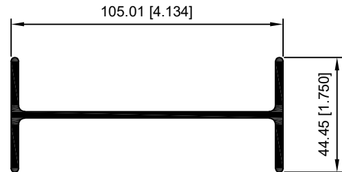
10047-PERFIL I DE 4" S/CEJA
