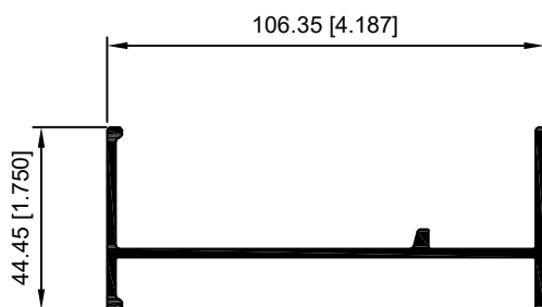
10043-PERFIL I DE 4.18"
