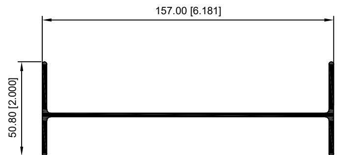
10035—PERFIL I LISO DE 6.16”
