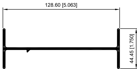
10014—PERFIL I PESADO P. 5 1/16 CON MUESCA
