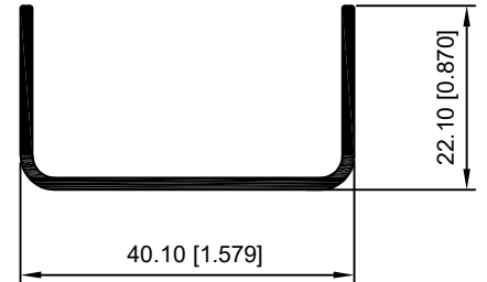
10001—CANAL EXTRA LIGERO
