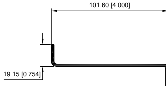
10007-PERFIL Z DE 4"
