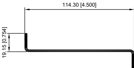
10008-PERFIL Z DE 4.5"
