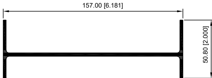
10045-PERFIL I 6" S/CEJA
