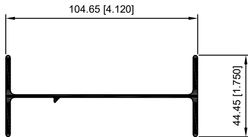
10012—PERFIL I PERALTE 4
