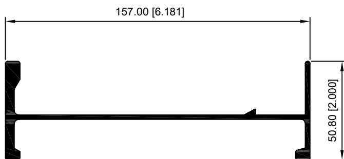
10034—PERFIL IR6 ALTERNATIVO
