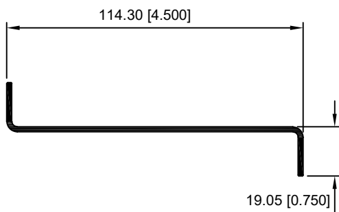
10018—PERFIL Z DE 4.5"
