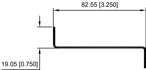
10000—PERFIL Z 3 1/4 EXTRA LIGERO
