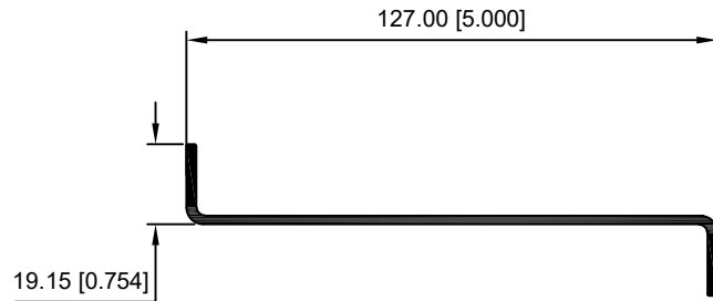
10009-PERFIL Z DE 5"
