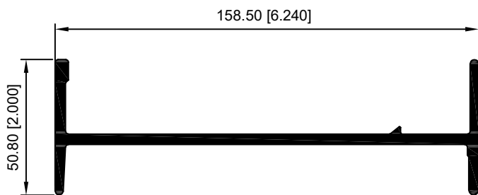
10041-PERFIL I SUPER PESADO P-6.240
