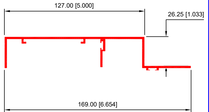
HEMBRA VERTICAL 40070
