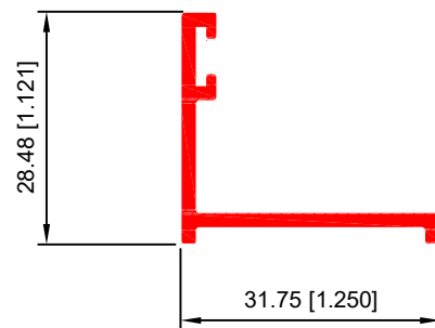
MARCO VENTILA 40092
