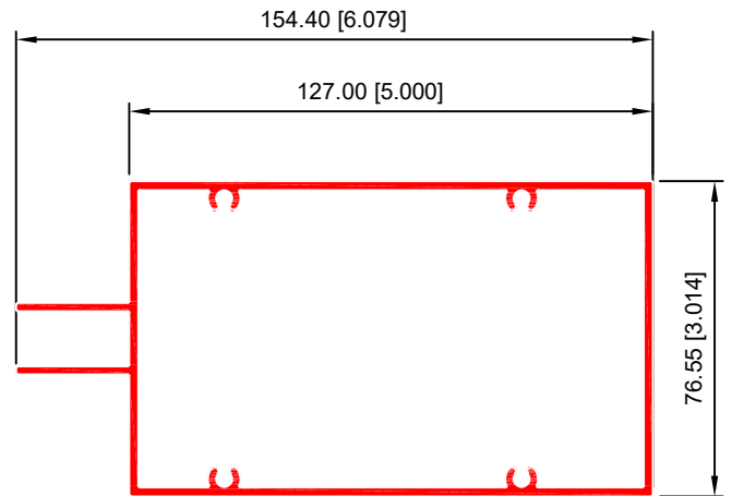
BASICO HORIZONTAL 40086
