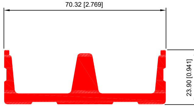
REFUERZO HORIZONTAL 40236
