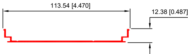
REFUERZO VERTICAL 40181
