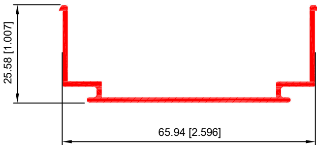
RFUERZO VERTICAL 40071
