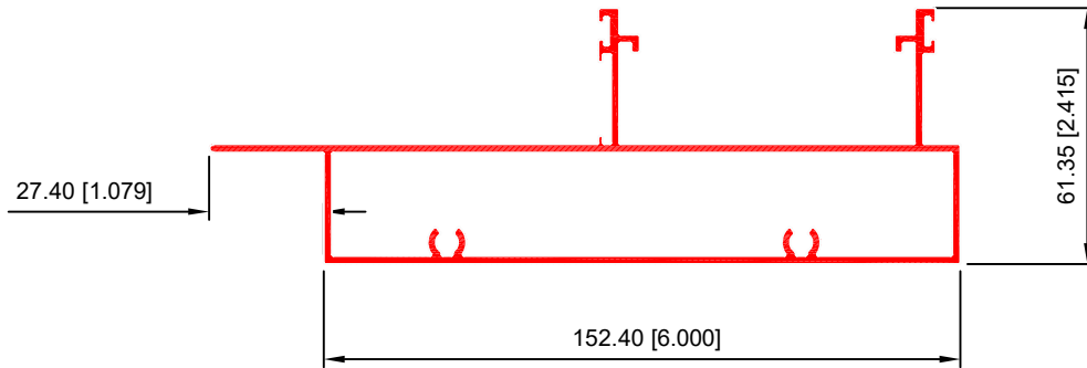
MACHO HORIZONTAL 40238
