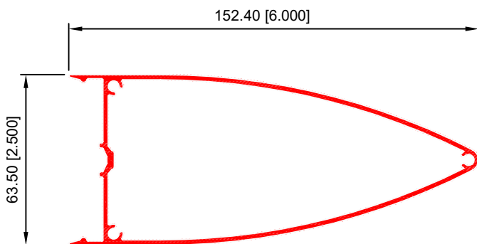
PARTELUZ DE 6" 40292
