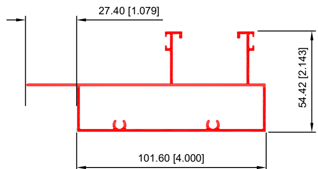
MACHO HORIZONTAL 40049
