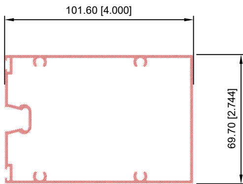
BASICO HORIZONTAL 40046
