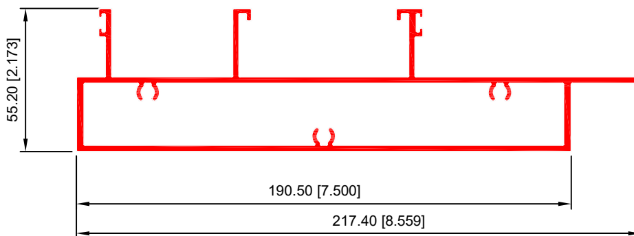
MACHO HORIZONTAL 40195
