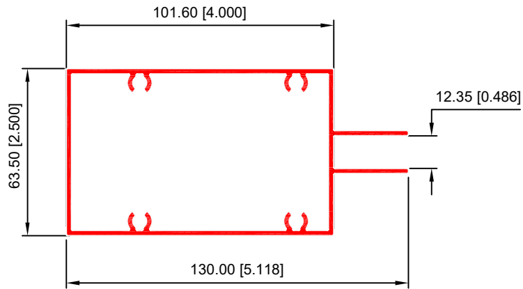
40018-BASICO HORIZONTAL
