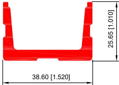
40044 REFUERZO HORIZONTAL
