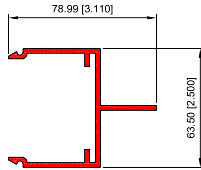
BASICO ABIERTO 40343
