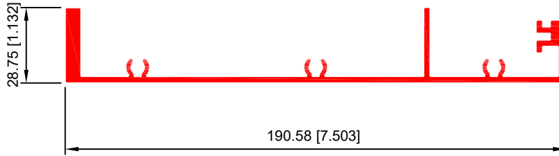
HEMбра HORIZONTAL 40196
