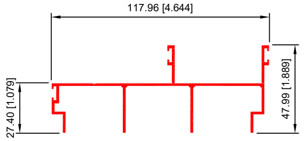
MACHO HORIZONTAL 40068
