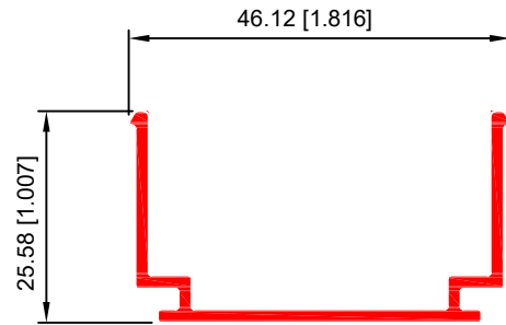
REFUERZO VERTICAL 40045
