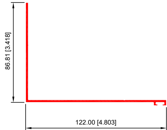
CUBRELOSA 40041
