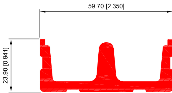
REFUERZO HORIZONTAL 40085
