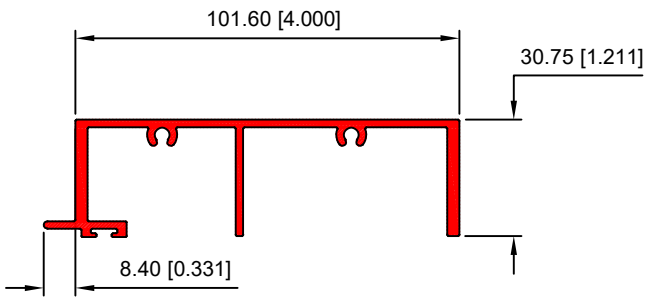
HEMBRA HORIZONTAL 40459
