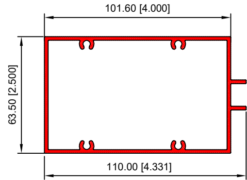
BASICO HORIZONTAL 40550
