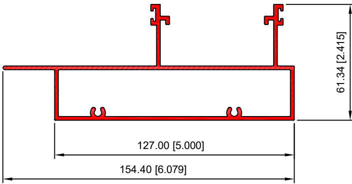
MACHO HORIZONTAL 40083
