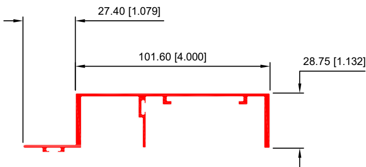
HEMBRA VERTICAL 40048
