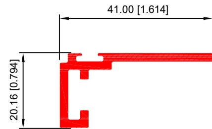
ADAPTADOR 40182
