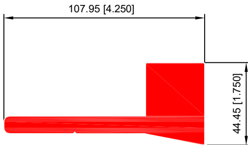
ANCLA 40052
