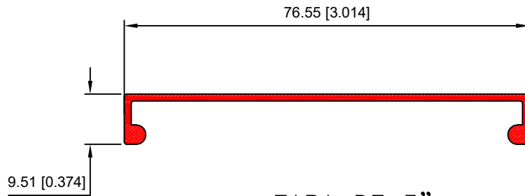
TAPA DE 3'' 40484
