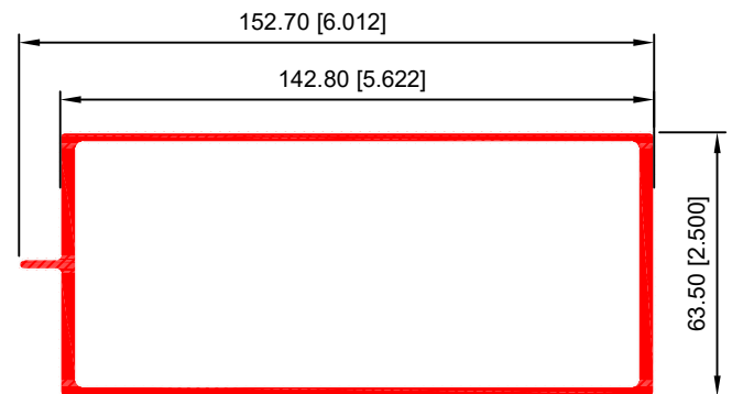
BASICO DE 5.6" 40335
