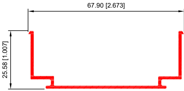
REFUERZO VERTICAL 40089
