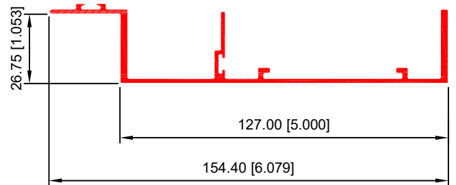
HEMBRA VERTICAL 40088
