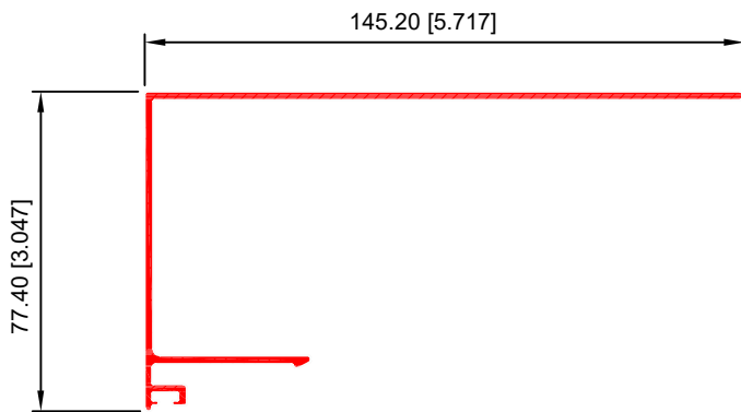
ZOCLO 40091
