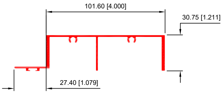
HEMBRA HORIZONTAL 40050
