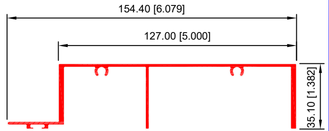
HEMBRA HORIZONTAL 40084
