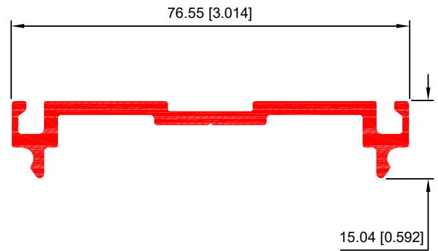
MULLION DE 3" 40127
