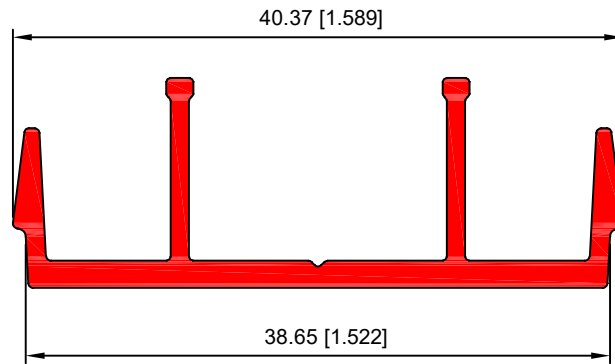
40573-TAPA PARTELUZ
