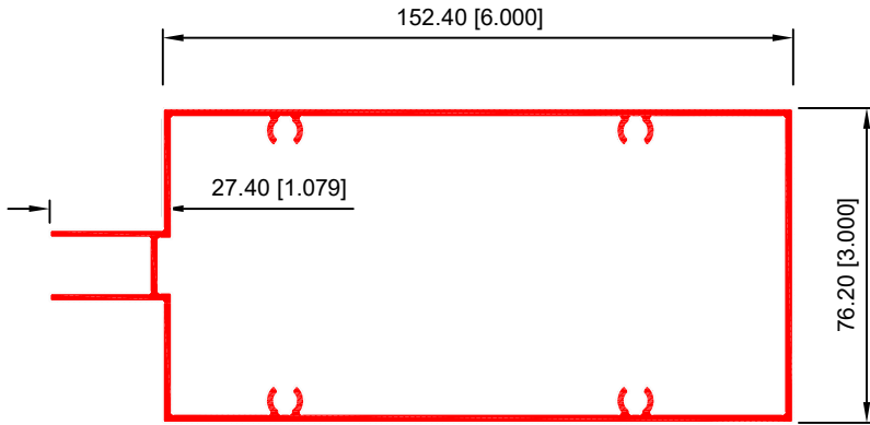
BASICO HORIZONTAL 40230
